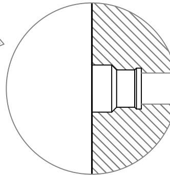
DETALHE (LUVAS ENGASTADA)
