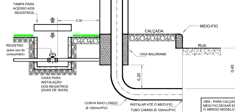
VISTA LATERAL EM CORTE
